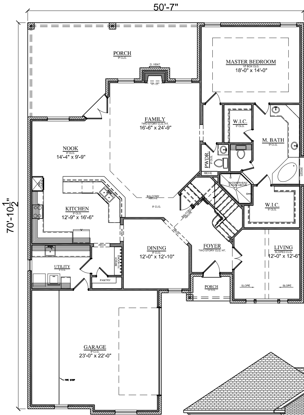
Floor Plan N.T.S.
