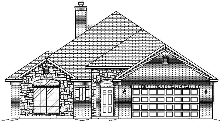
Front Elevation N.T.S.
